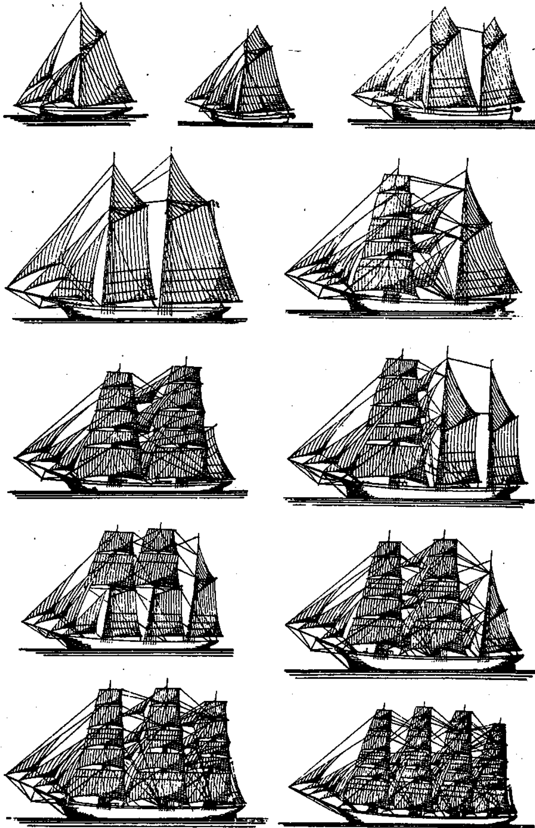
Skeppstyper: 1 raden: slup(kutter), jakt, galeas 2 raden: fore-and-aft skonert, skonert 3 raden: brigg, skonertskepp 4 raden: skonertbark, bark 5 raden: fullriggare, fyrmastad fullriggare
