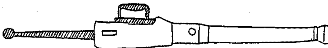
Brede Ullekanon nr 2 med svans och löstagbart kammarstycke som det bör ha sett ut enl. Guilmartin: Gunpowder and Calleys 1976.
