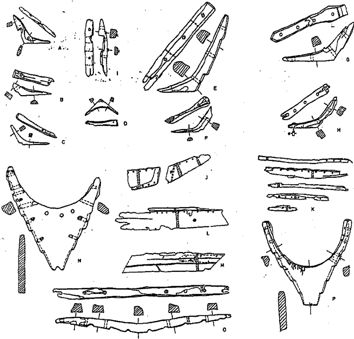
Fynd av skeppsdetaljer från åbrådden av Fribrødre å på Falster. Efter Jan Skamby Madsen, Vikingeskibshallen, Roskilde.
