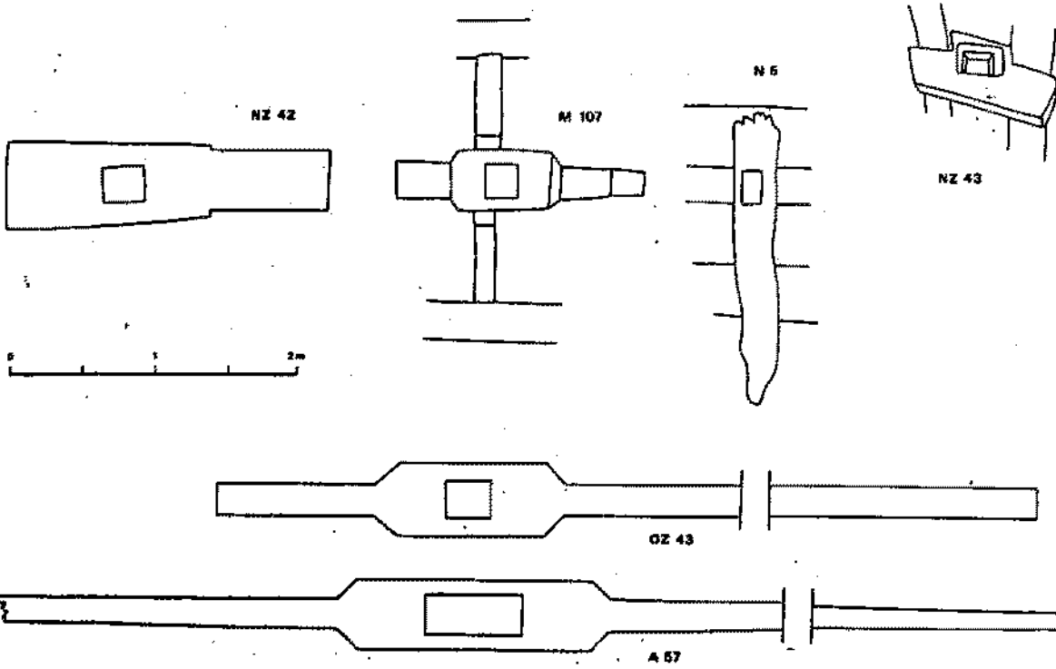
Mastställning/kölsvin i holländska koggfynd (Reinder Reinders) Nedan Bremerkoggen som jämförelse i en tvärsektion mot stäven.
