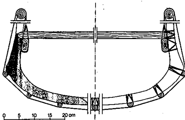
En tänkbar tvärsektion i en skinnbåt med Husumhornet som spant. Efter Ellmers.
