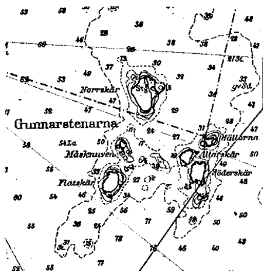
ur sjökort 715:a
