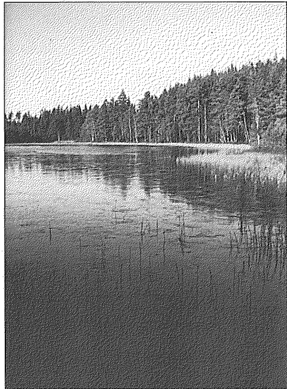
Lillegölen är en liten sjö belägen långt inne i skogen i södra Ydre, Östergötland. Foto: Johan Rönnby.
