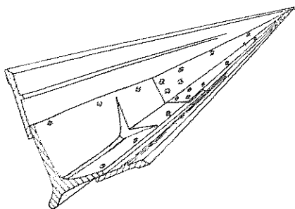
Detalj av Björkebåtens stävkonstruktion. Ritning ur Humbla 1948.
